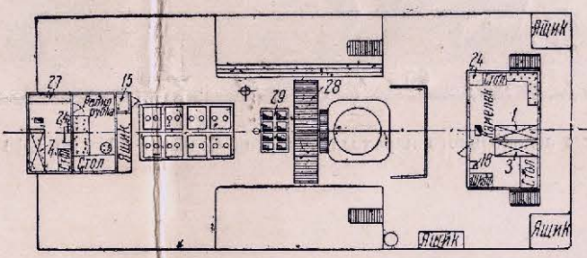
Поперечный разрез и план палуб ледокольного парохода „Георгий Седов“
