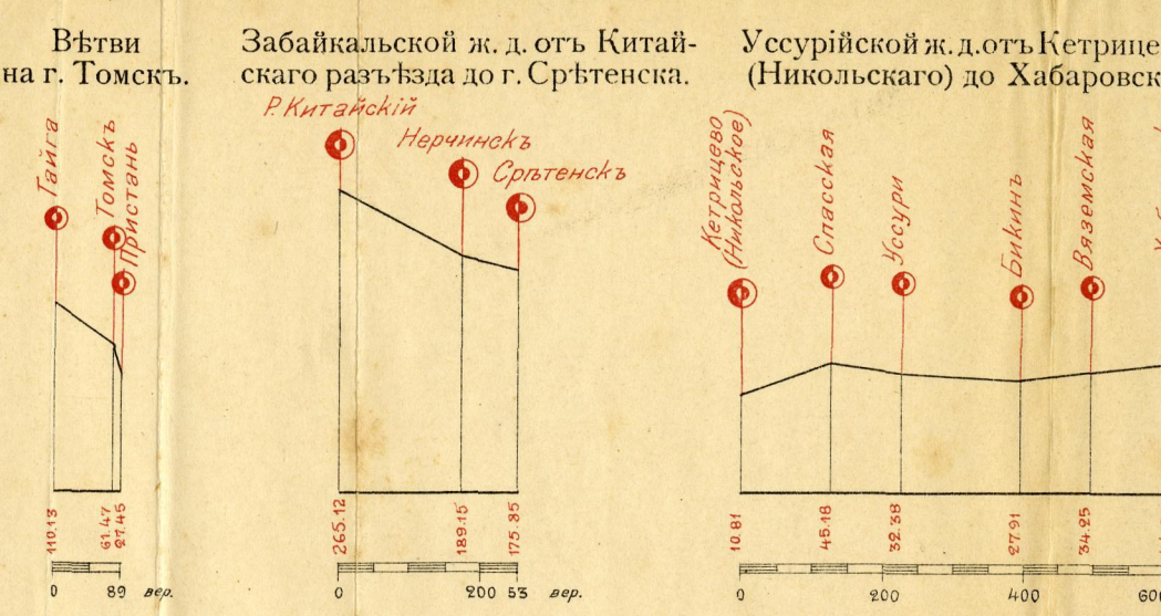
Сокращенный профиль и графикъ хода укладки пути.
