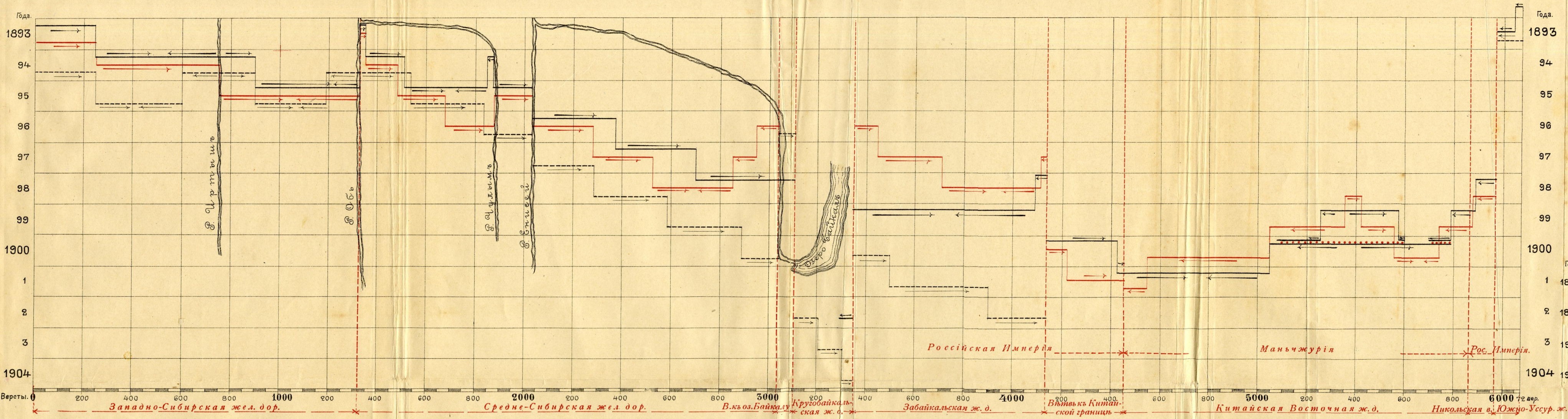
Графикъ хода укладки сплошного рельсового пути от Челябинска до Владивостока.
